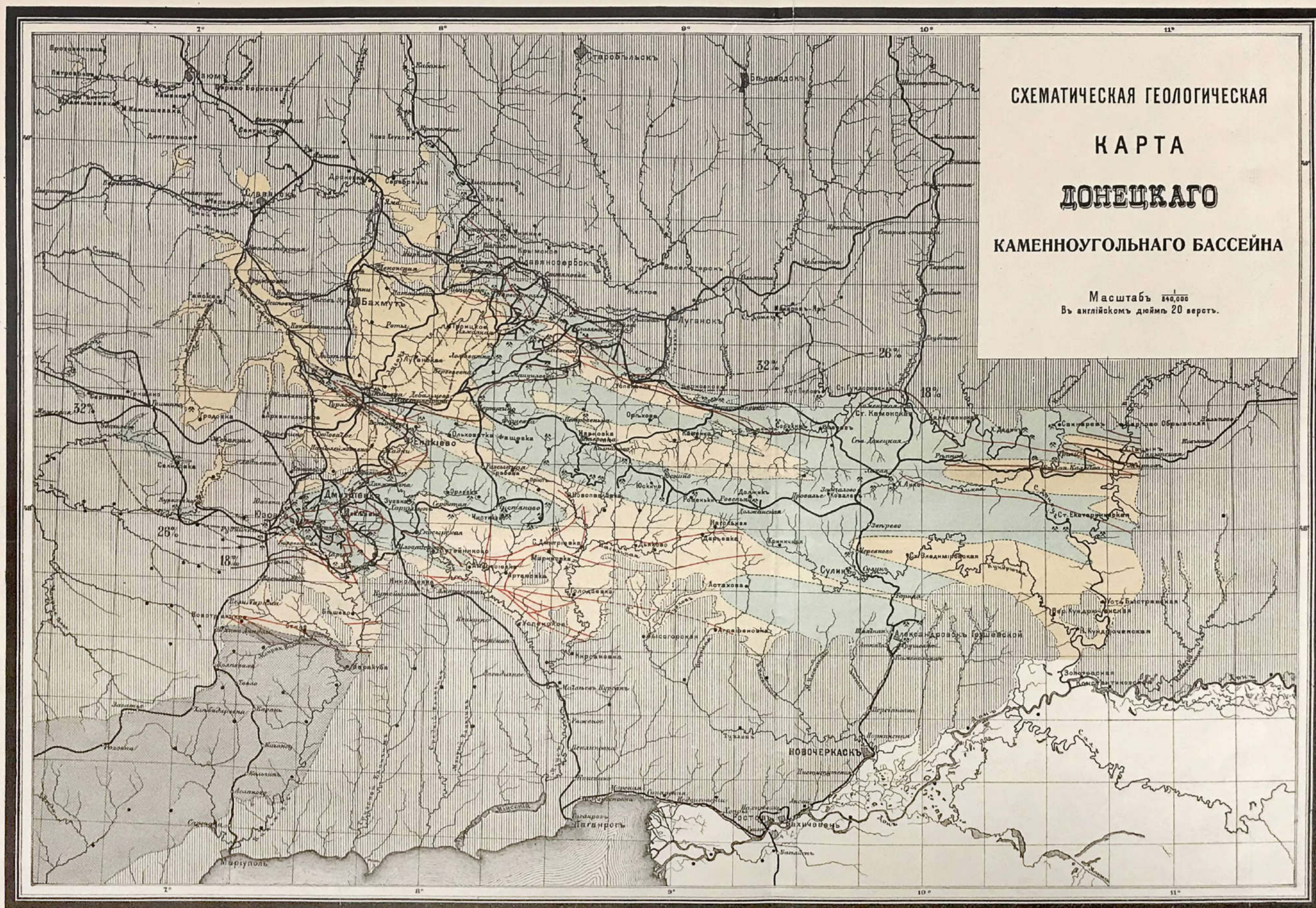
Схематическая геологическая карта Донецкого каменноугольного бассейна.
